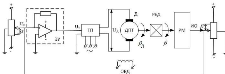
Рис. 1. Электромеханическая следящая система с потенциометрическим измерительным устройством
